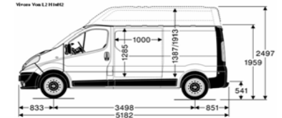
Vivaro Van L2 H146Z
