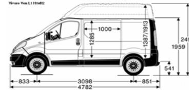
Vivaro Van L1 H146Z
